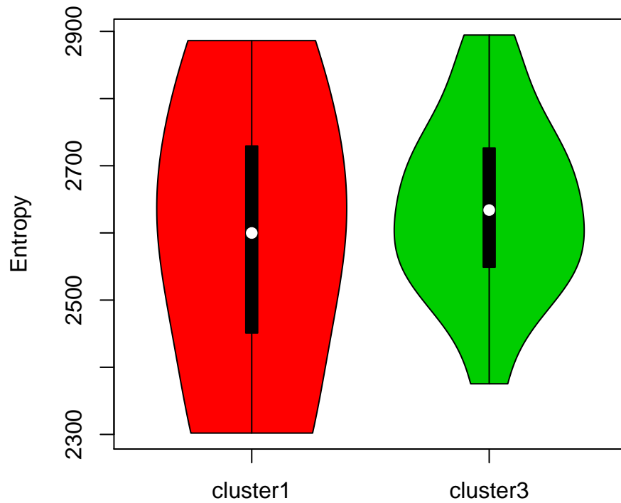
Cluster Entropies
